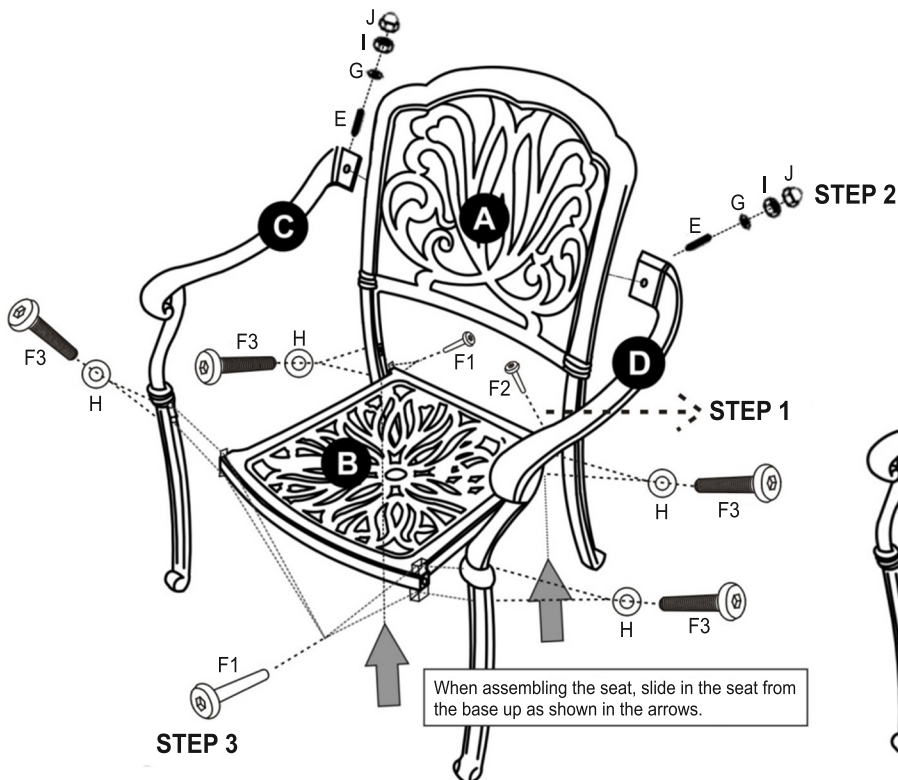
F1 8pcs M6x40mm
